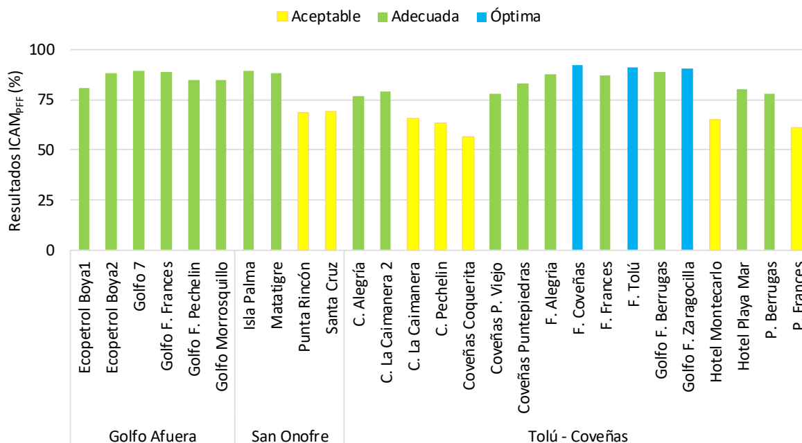
Figura 9.4. Calidad del agua superficial según el ICAM PFF en las estaciones marinas y costera en el departamento de Sucre, en el muestreo del segundo semestre de 2018.
