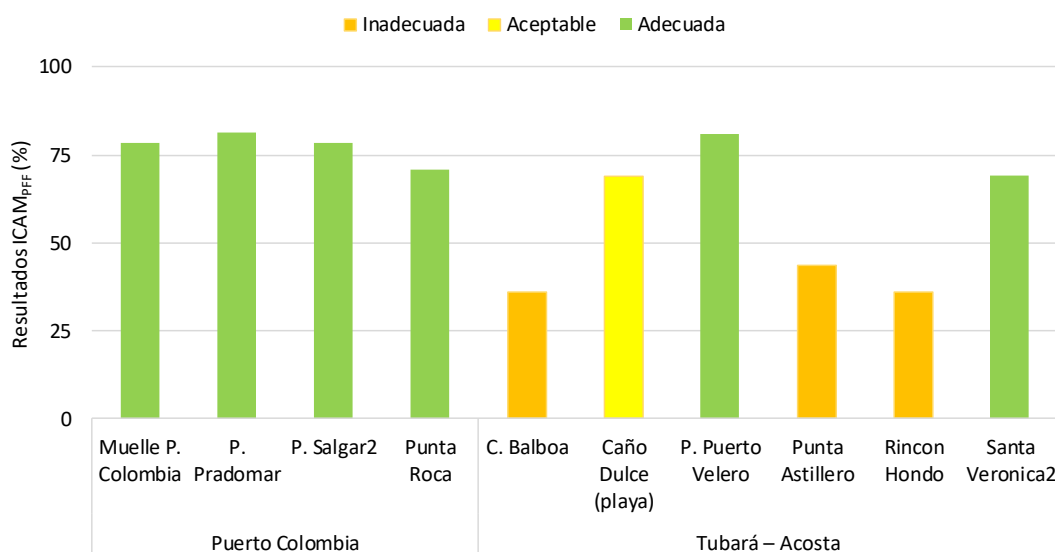
Figura 7.4. Calidad de agua superficial según el ICAM PFF en las estaciones marinas y costeras en el departamento de Atlántico, en el muestreo del segundo semestre de 2018.
