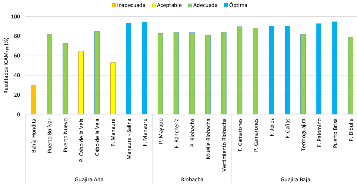
Figura 5.5. Calidad del agua superficial según el ICAM PFF en las estaciones marinas y costera del departamento de La Guajira, en el muestreo REDCAM del primer semestre de 2019.
