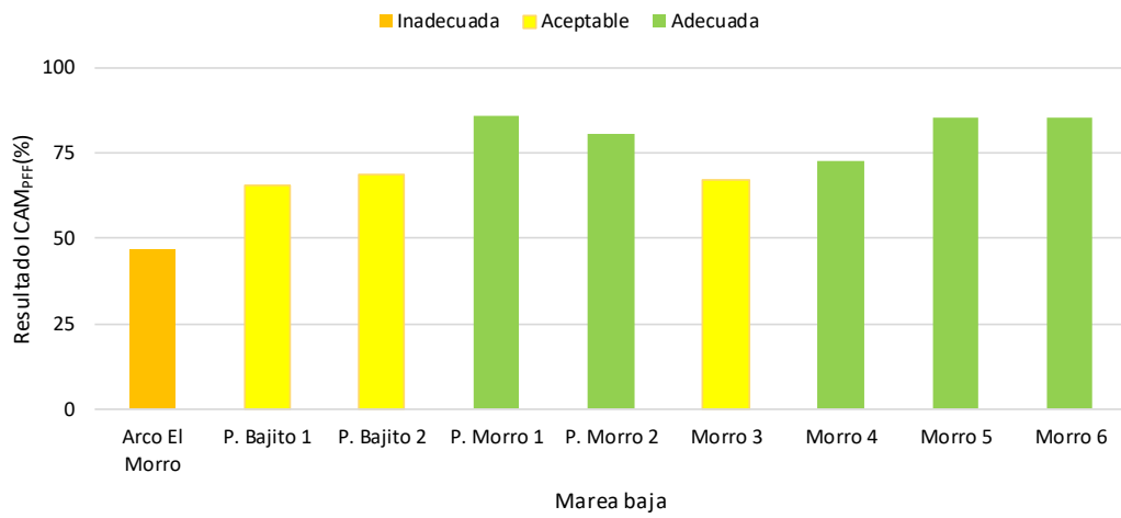
Figura 15.4. Calidad del agua superficial según el ICAM PFF en las estaciones marinas y costera en el departamento de Nariño, en condiciones de marea alta (a) y marea baja (b) en el muestreo del primer semestre de 2019.
