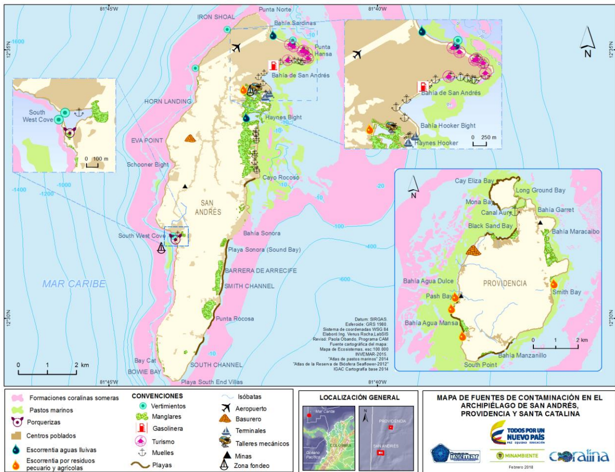
Figura 4.3. Mapa de la distribución de ecosistemas marino-costeros, centros poblados, actividades antropogénicas y fuentes terrestres y marinas de contaminación en las Islas de San Andrés, Providencia y Santa Catalina, Caribe colombiano
