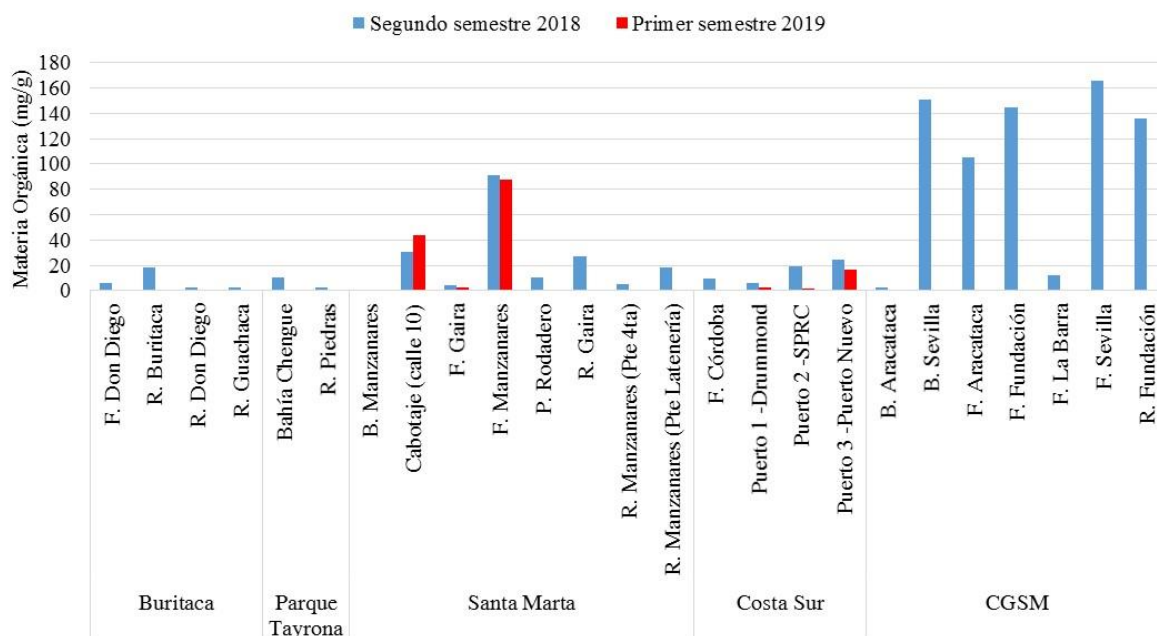
Figura 6.6. Contenido de materia orgánica oxidable en los sedimentos de las estaciones REDCAM en el Magdalena, medidos en los muestreos del segundo semestre de 2018 y primer semestre de 2019.
