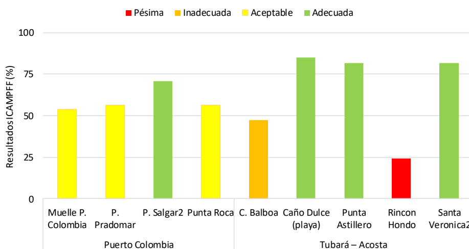
Figura 7.5. Calidad de agua superficial según el ICAM PFF en las estaciones marinas y costeras en el departamento de Atlántico, en el muestreo del primer semestre de 2019.
