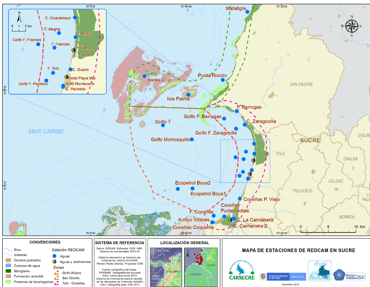
Figura 9.1. Mapa con las estaciones de muestreo de la REDCAM en el departamento de Sucre. Los puntos azules indican las estaciones de muestreo de agua superficial, y los puntos bicolor (azul y marrón) corresponden a estaciones donde se muestrea agua y sedimento. Los polígonos punteados enmarcan las zonas de muestreo.
