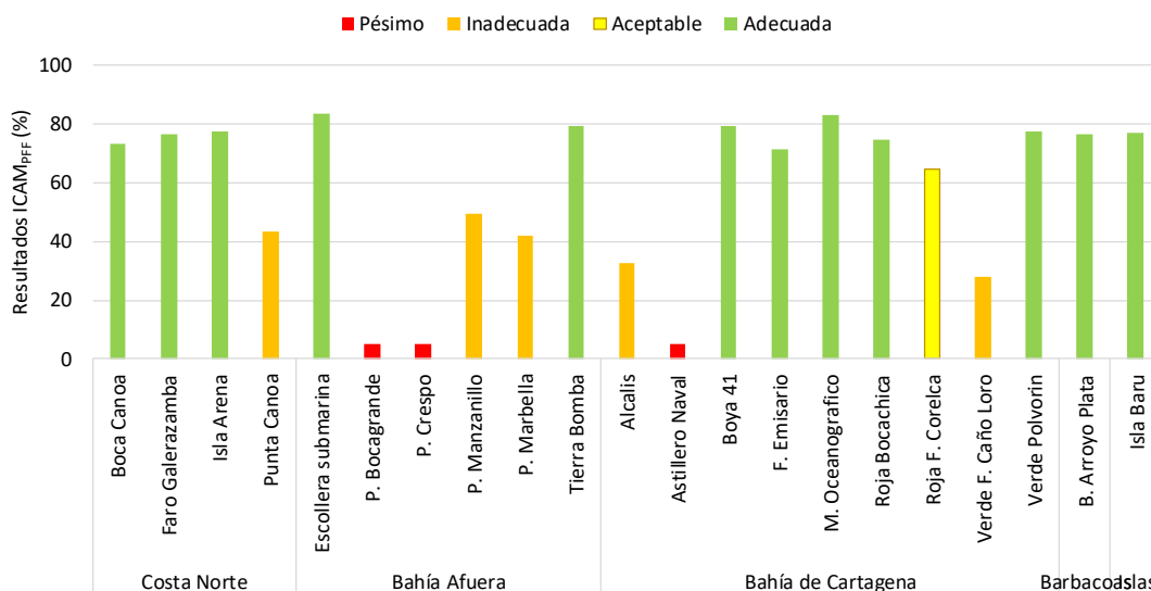
Figura 8.4. Calidad del agua superficial según el ICAM PFF en las estaciones marinas y costera del departamento de Bolívar, en el muestreo del segundo semestre de 2018.
