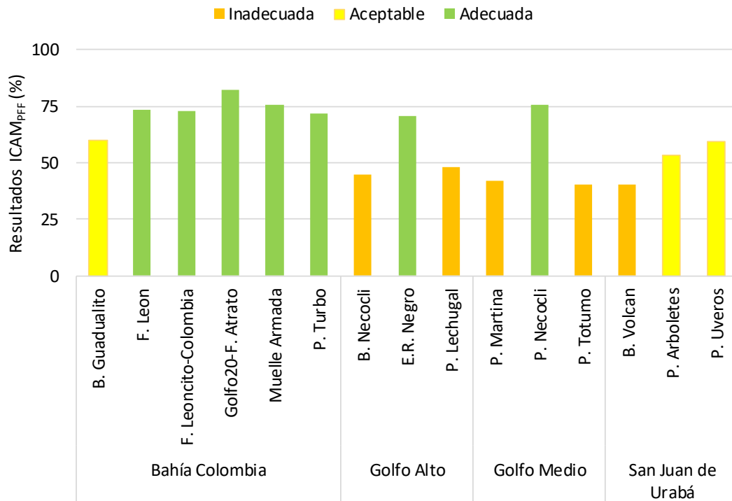
Figura 11.4. Calidad de agua superficial según el ICAM PFF en las estaciones marinas y costeras en el departamento de Antioquia, en el muestreo del segundo semestre de 2018.
