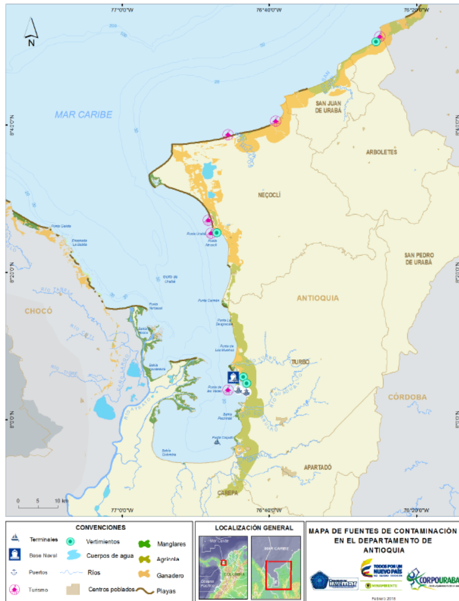
Figura 11.3. Mapa de la distribución de ecosistemas marino-costeros, centros poblados, actividades antropogénicas y fuentes terrestres y marinas de contaminación en el departamento de Antioquia, Caribe colombiano.
